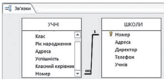
Рис. 4. Зв'язок між таблицями типу 1 : ∞
